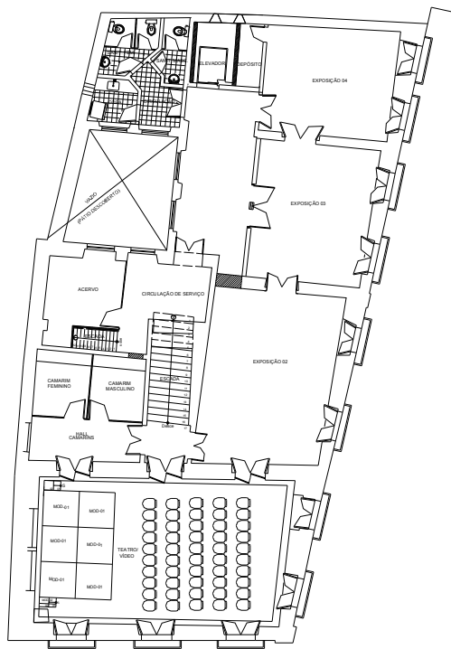
PLANTA BAIXA - 1º PAVIMENTO ÁREA CONSTRUTIVA: 8.040m²
