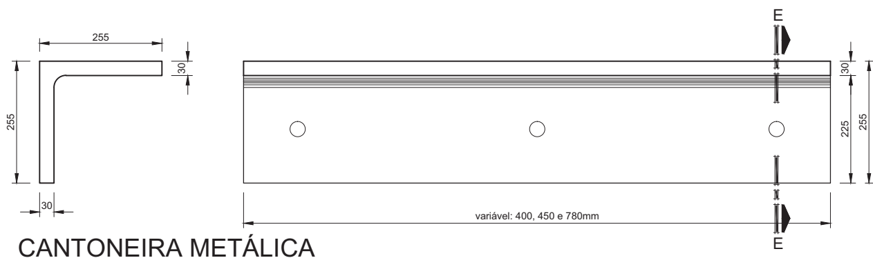
CORTE F-F
