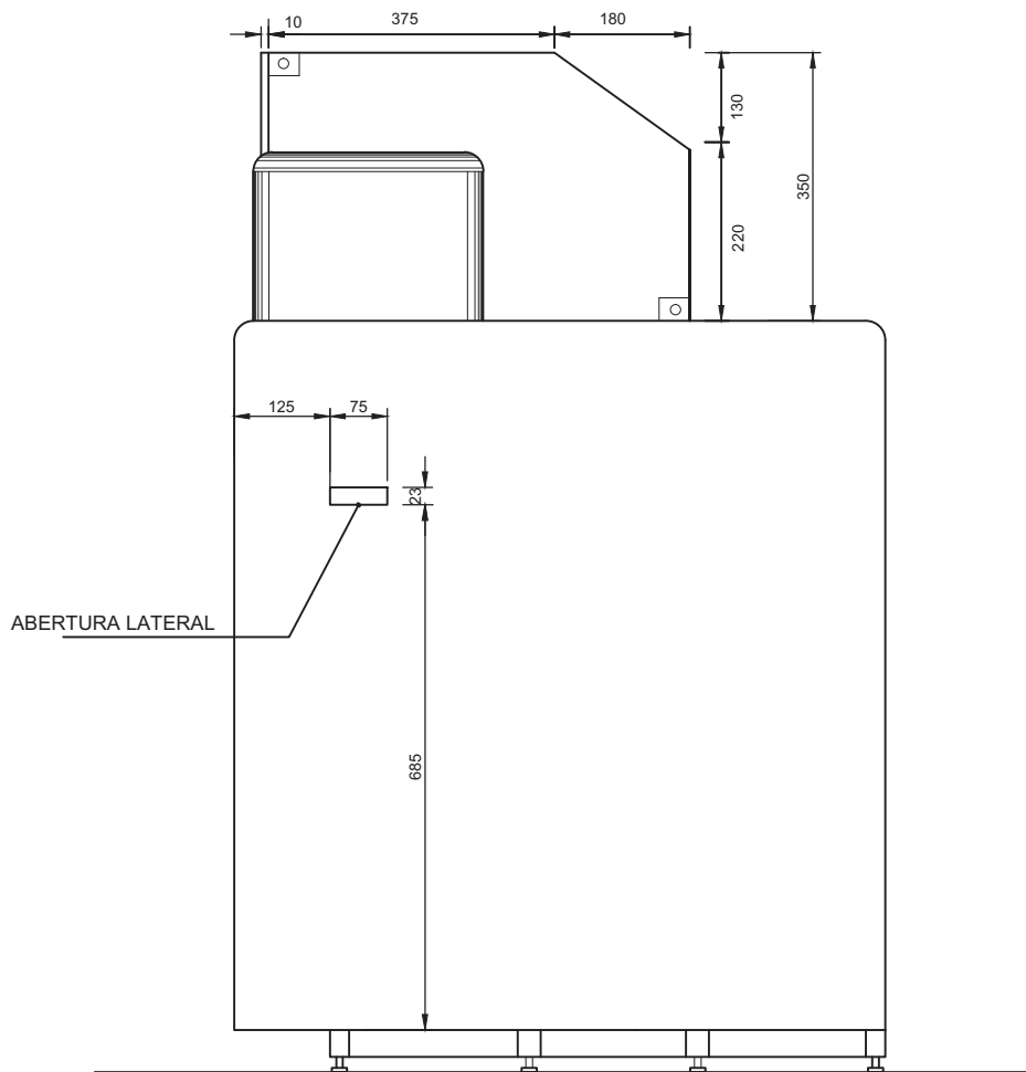
VISTA LATERAL
